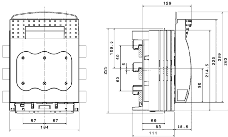
141A-NFJ200C
