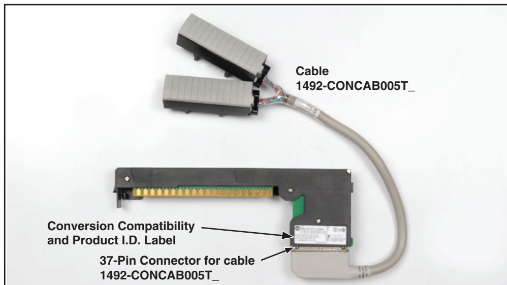
1492-CM1771-LA004 Conversion Module
