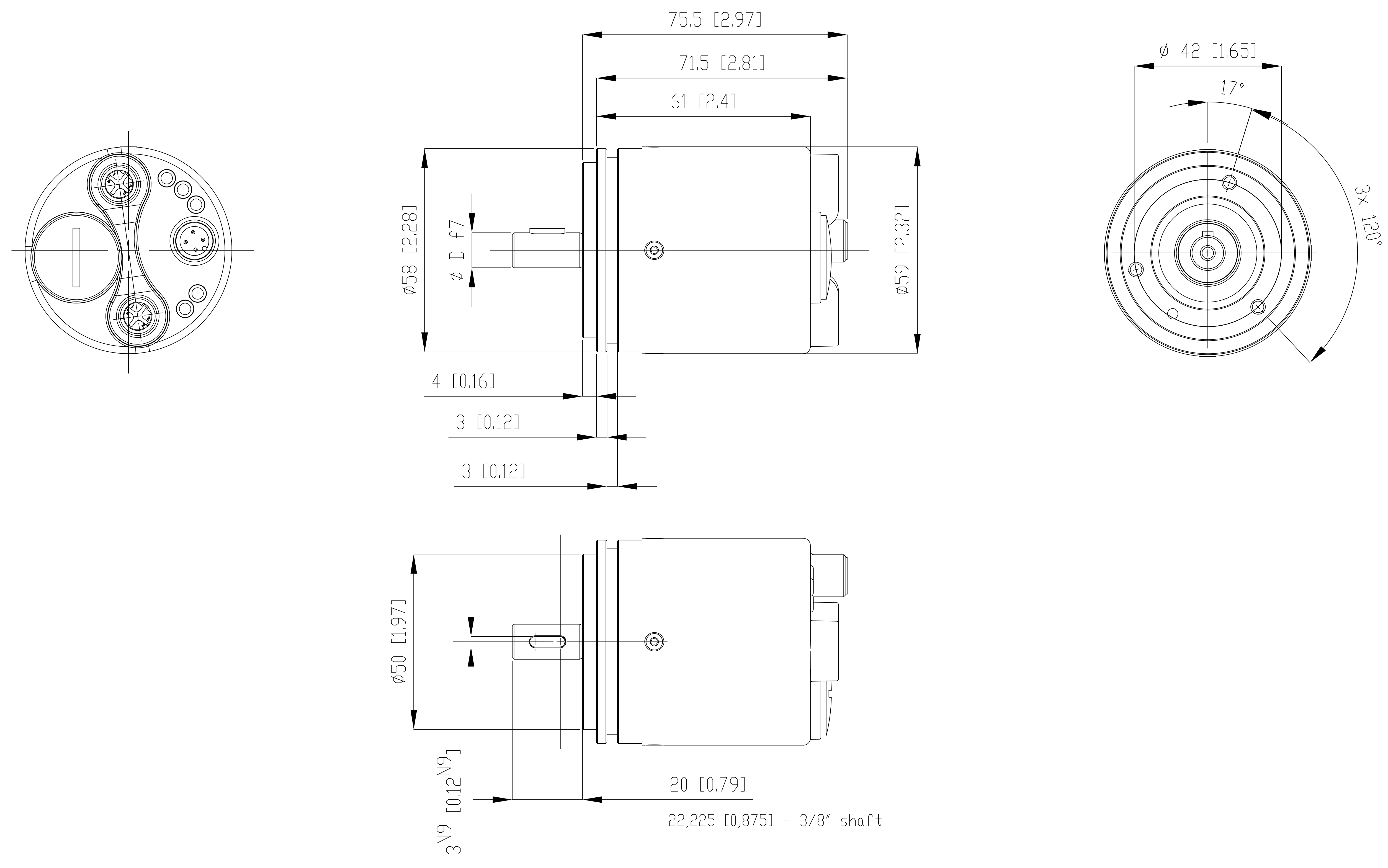
SYNCHRO FLANGE
